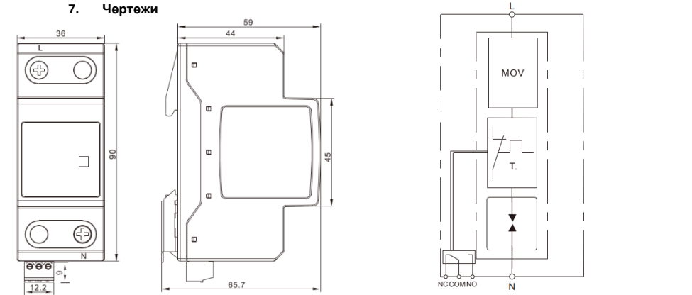
Рис.3. Габаритный чертеж
