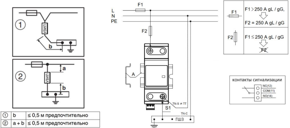
Рис.1. Варианты подключения
