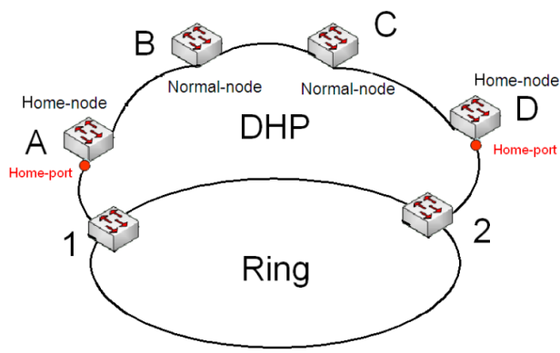
Рис. 192. DHP
