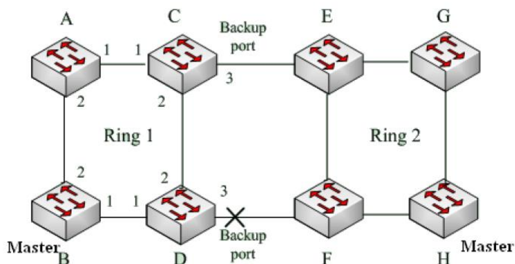
Рис. 183. ST-RING+ топология
