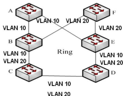
Рис. 182. ST-RING-VLAN
