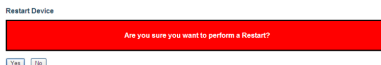
Рис. 8. Перезагрузка
