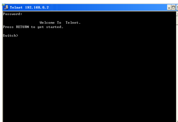
Рис. 7. Интерфейс telnet
