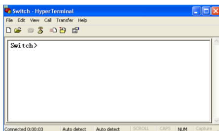
Рис. 5. CLI
