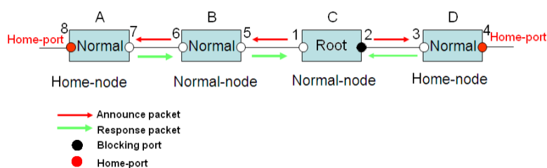
Рис. 193. Конфигурация DHP
