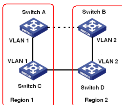
Рис. 203. MSTP топология
