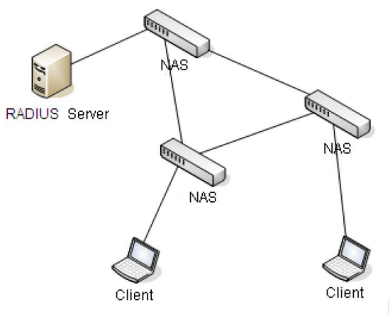
Рис. 118. Radius структура
