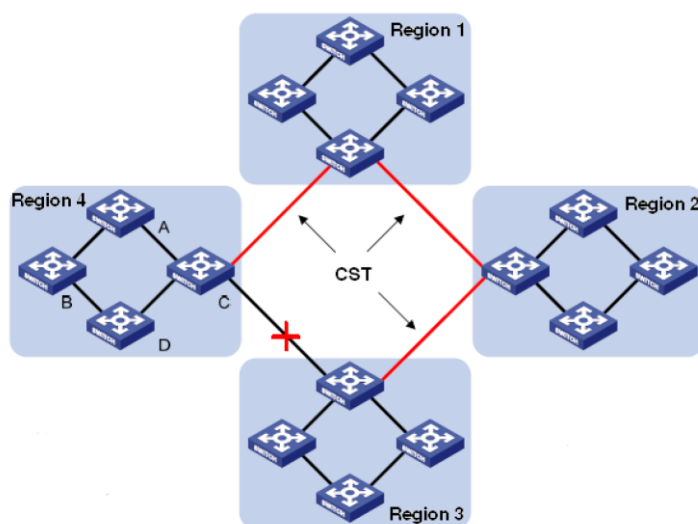
Рис. 204. MSTP концепт
