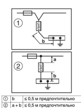
Рис.1. Варианты подключения
