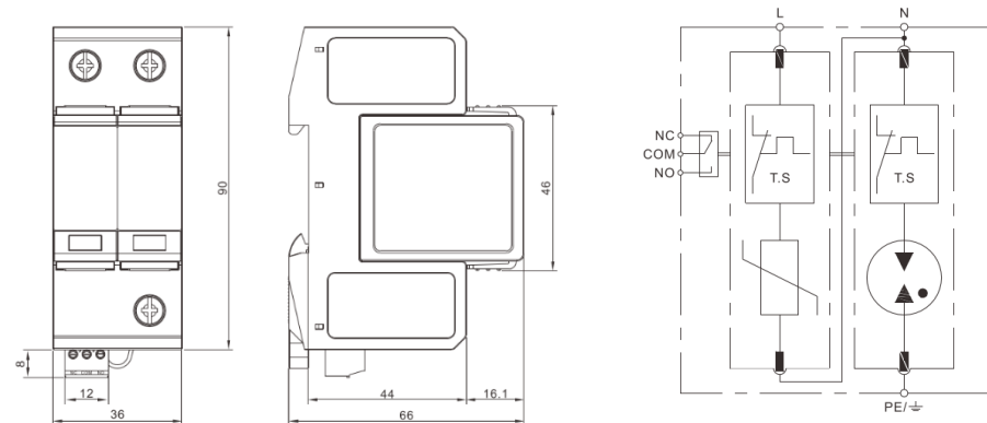
Рис.3. Габаритный чертеж
