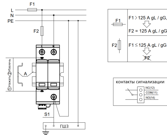
Рис.2. Схема подключения
