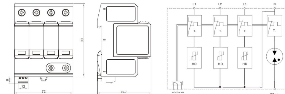
Рис.3. Габаритный чертеж
