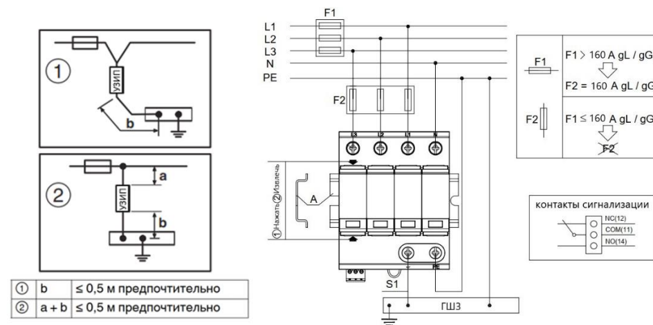
Рис.1. Варианты подключения
